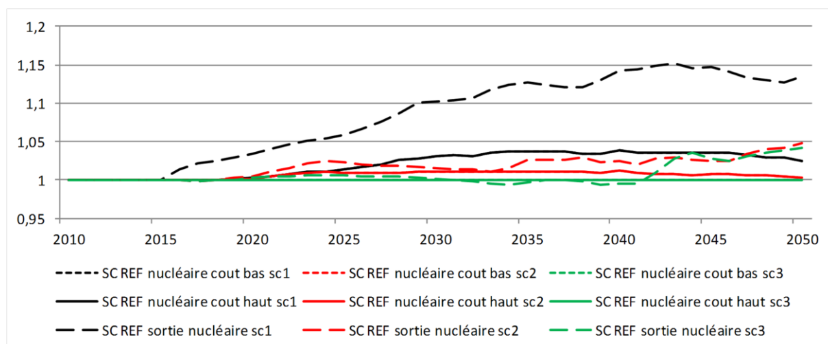
Figure 3 : Budget énergie des ménages entre 2010 et 2050 dans les scénarios de référence en fonction du rythme de déclasséement des centrales nucléaires et du nouveau nucléaire (coût élevé, bas ou sortie du nucléaire) en indice par rapport au scénario de prolongation de la durée de vie de toutes les centrales avec coût bas de l'EPR
